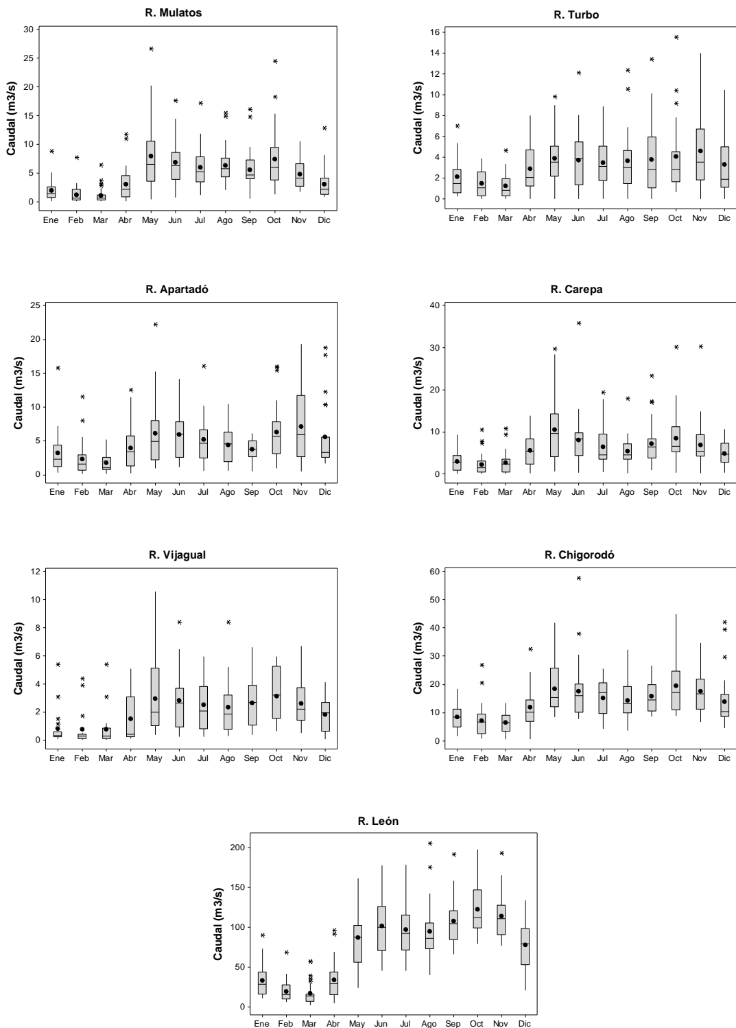
Figura 2. Variabilidad intra-anual del caudal (m 3 /s) en las cuencas de los ríos Mulatos, Turbo, Apartadó, Carepa, Vijagual, Chigorodó y León. Se indican las medias, los valores máximos y mínimos, y el intervalo de confianza del 95%.
