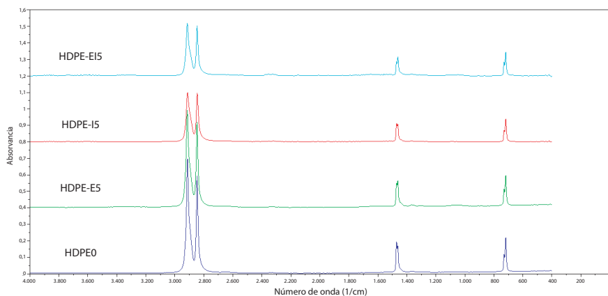
Figura 2. Espectros FTIR para el HDPE-GI sin reprocesar (HDPE0), extruido 5 veces (HDPE-E5), inyectado 5 veces (HDPE-I5) y extruido/inyectado en 5 ciclos (HDPE-EI5).
