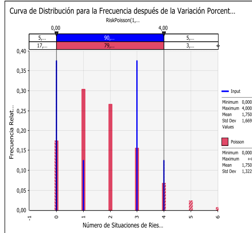
Datos para las curvas distribución finales de frecuencia y severidad de los EPC
