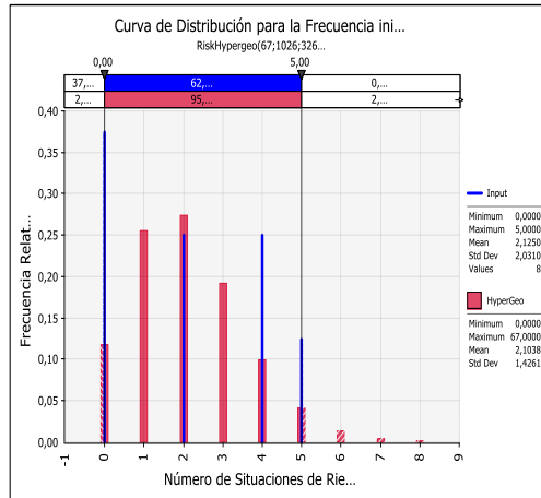
Datos para las curvas de distribución iniciales de frecuencia y severidad de EPC
