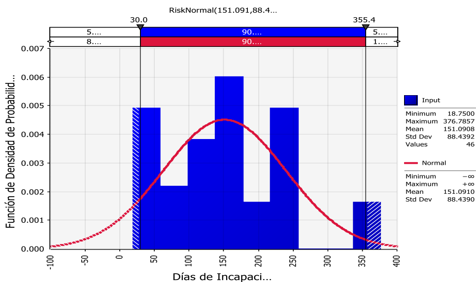
Figura 50. Curva de distribución de la severidad. Elaborada por el Autor
