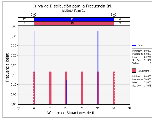
Datos para las curvas de distribución iniciales de frecuencia y severidad de los EPC
