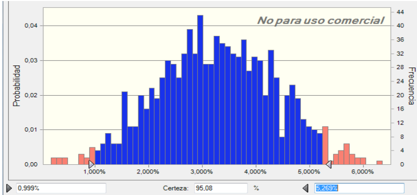
Ilustración 4 Distribución de Probabilidad de la serie de tiempo
