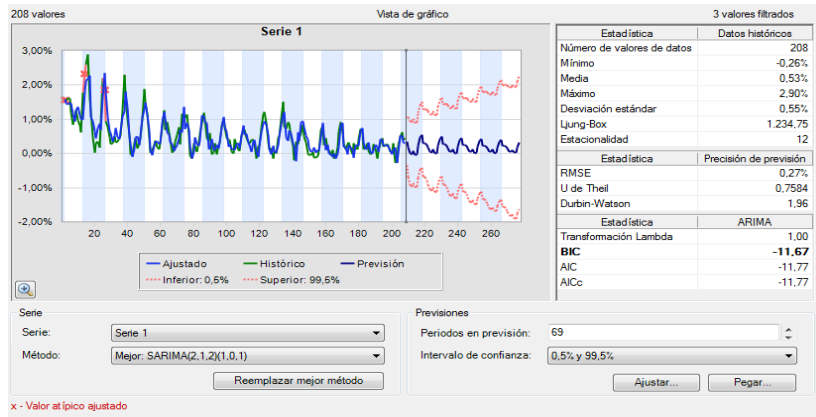
Ilustración 5. Ajuste y Selección del modelo
